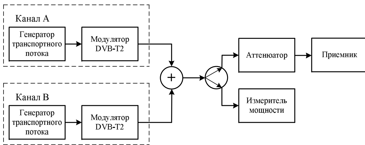
Рисунок 3 – Схема проверки 3
