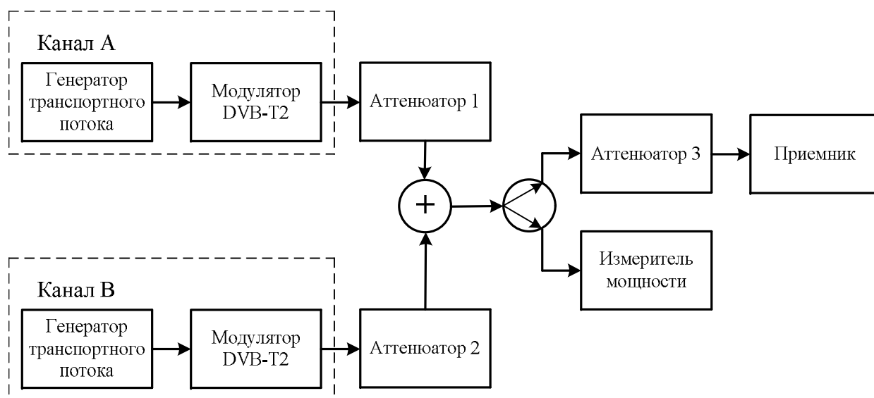
Рисунок 4 – Схема проверки 4
