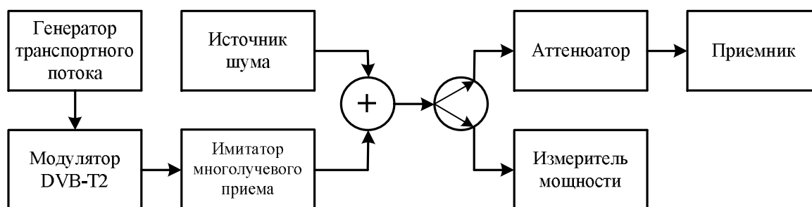
Рисунок 2 – Схема проверки 2
